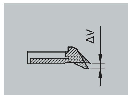
Předpětí
